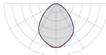
Curva fotometrica
